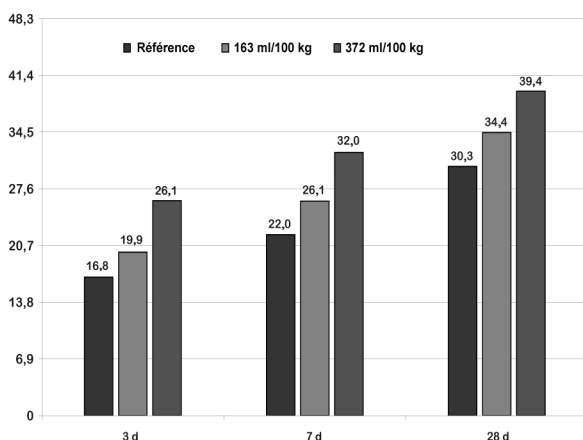
Résistance à la compression de PLASTOL 341 (MPa)
