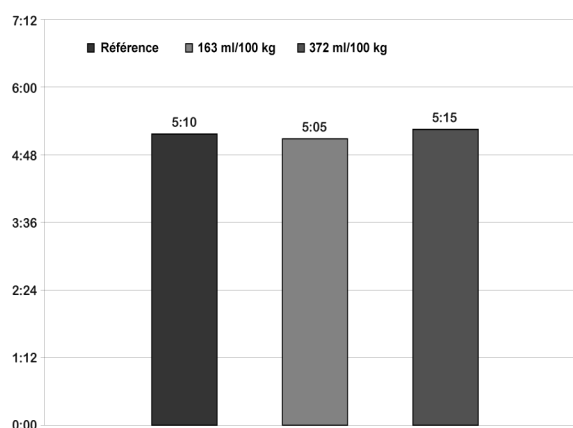
Temps de prise de PLASTOL 341 (h:min)
